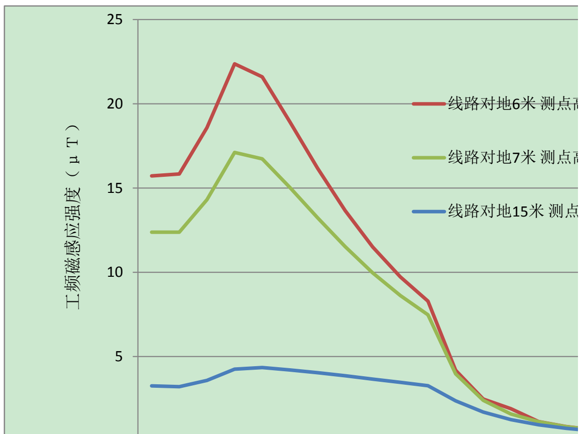
图 4 110kV 输电线路单回运行时工频磁感应强度变化趋势图
