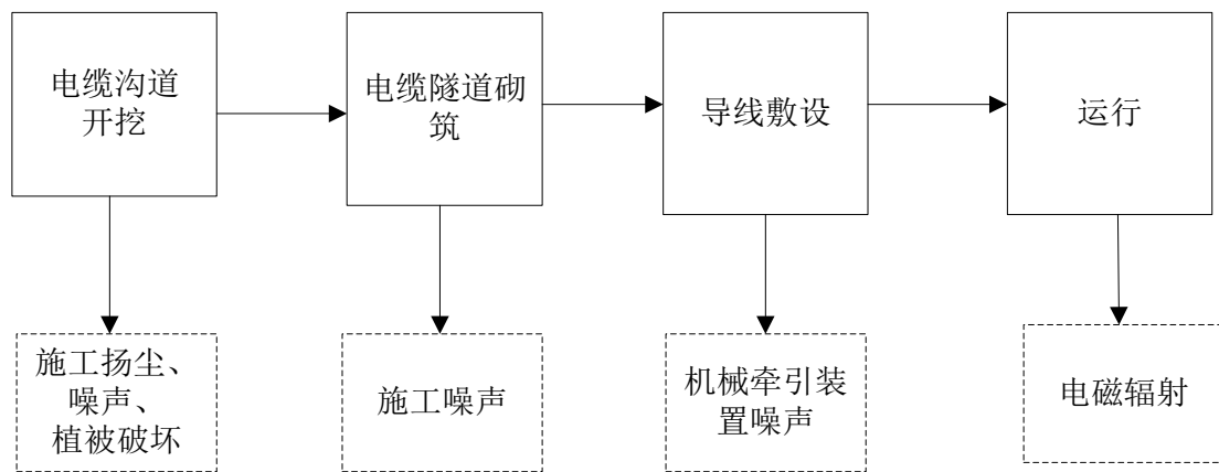
图 5-2 地下电缆工艺流程及产污环节示意图
