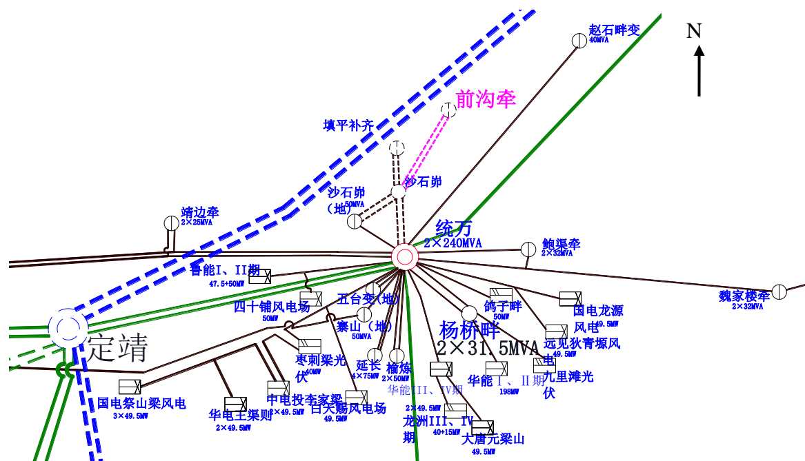
图 1-2 前沟牵地理接线图
