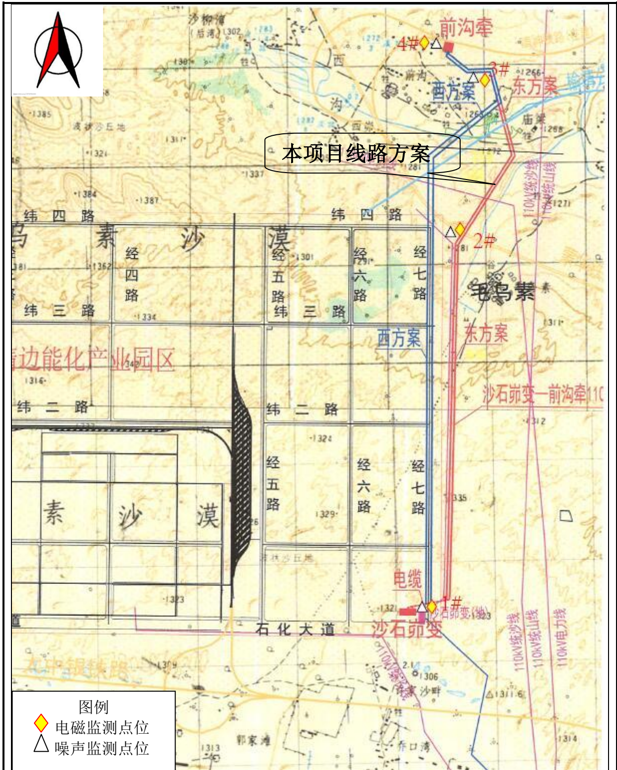
图 1-7 本项目线路路径及监测布点示意图
