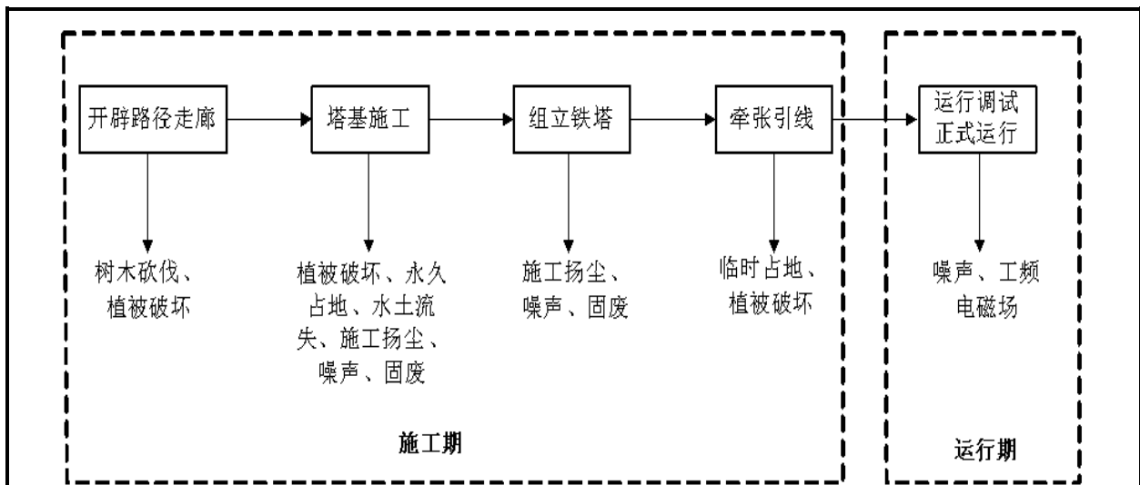
图 5-1 架空线路工艺流程及产污环节示意图
