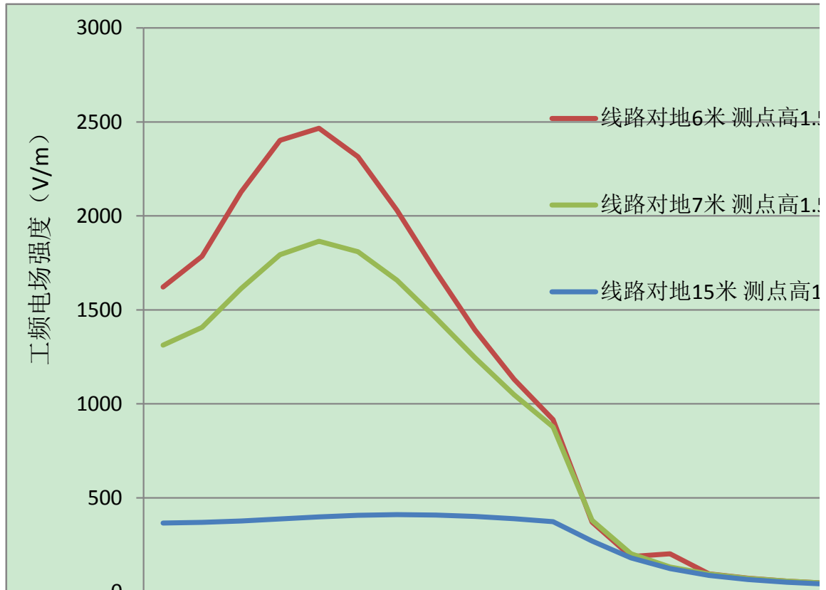
图3 110kV 输电线路单回运行时工频电场强度变化趋势图
