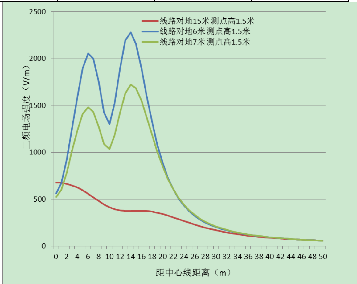
图 5 110kV 输电线路单回两塔并行运行时工频电场强度变化趋势图
